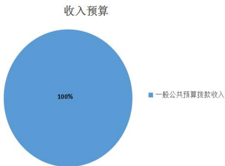
图 1：收入预算
